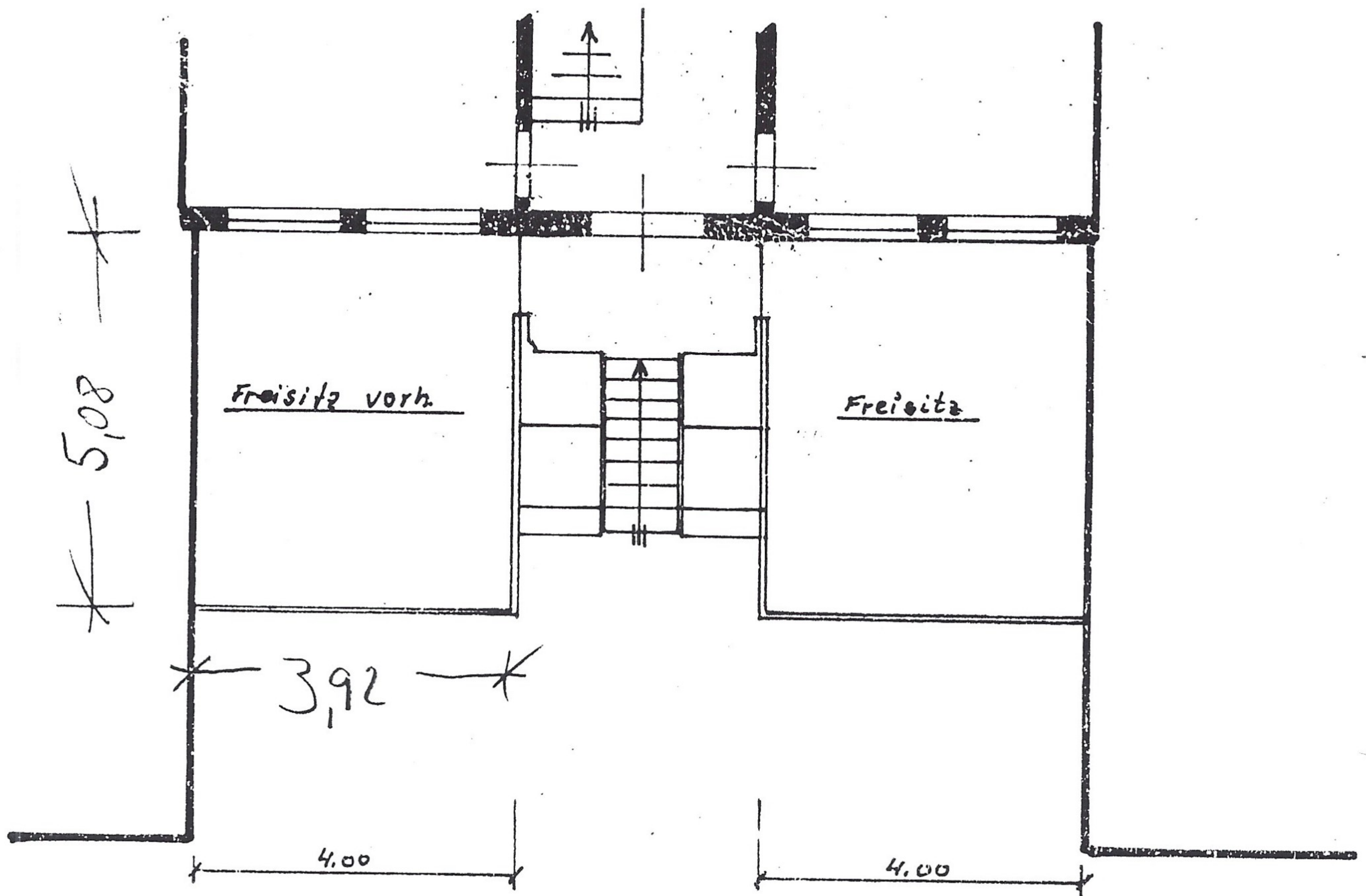
Grundriß
